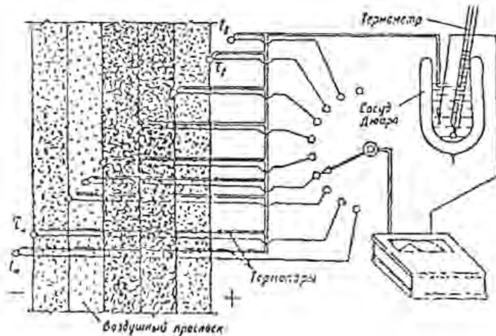
Рис. 10.7. Схема размещения датчиков термомпар при измерении температур в толще многослойного ограждения
