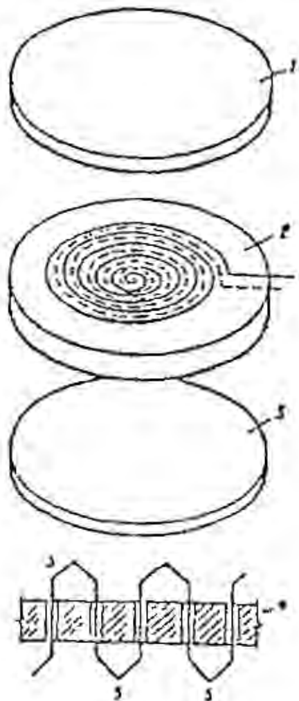
Рис. 10.5. Схема устройства тепломера З.З. Альперовича
