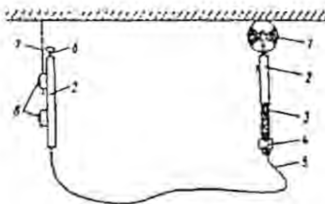
Рис. 5.4. Прогибомер П-1
