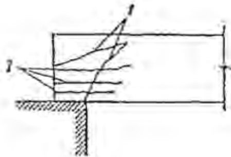
Рис. 6.5. Трещины в опорной части предварительно напряженного элемента
