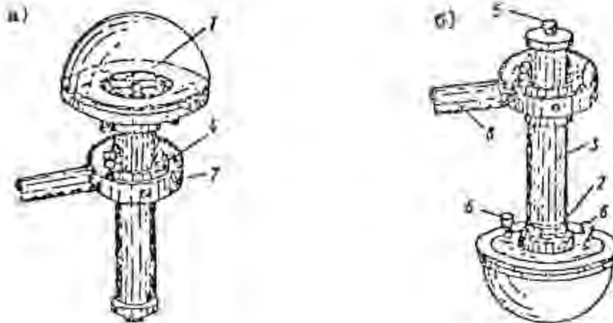
Рис. 10.4. Альбедометр
