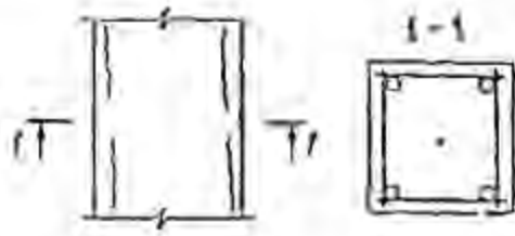
Рис. 6.3. Трещины вдоль продольной арматуры в сжатых элементах
