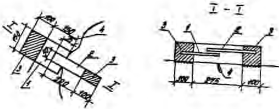
Рис. 5.7. Пластинчатый маяк из двух окрашенных пластинок
