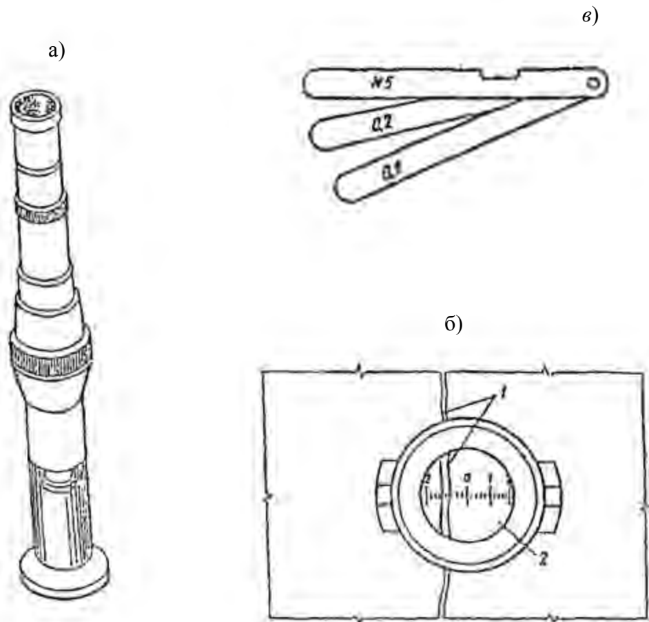
Рис. 5.5. Приборы для измерения раскрытия трещин
