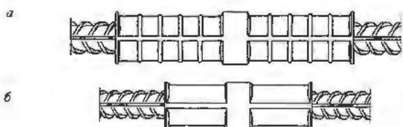
Рисунок Н.1 - Опрессованный стык построечного изготовления, произведенный на мобильном оборудовании многократным поперечным деформированием соединительной муфты с прожежками (а) и без прожежков (б)
